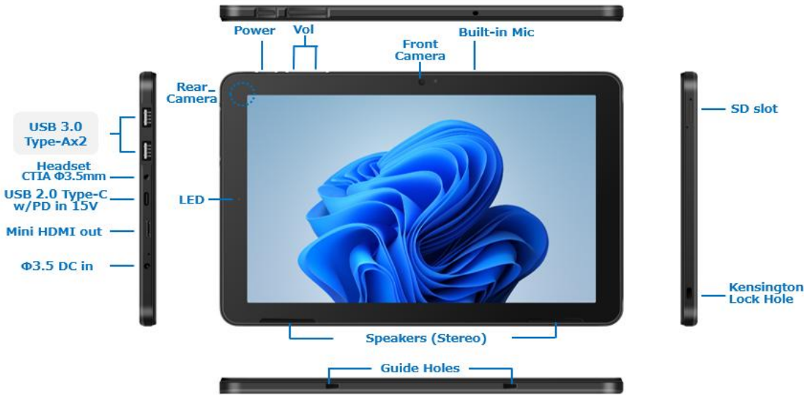
インターフェース配置図
